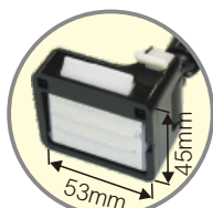
強力磁座
